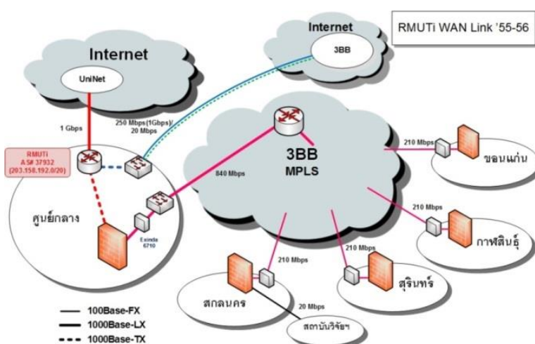
ภาพที่ 2 – 1 แผนผังการเชื่อมต่อเครือข่ายมหาวิทยาลัยเทคโนโลยีราชมงคลอีสาน
