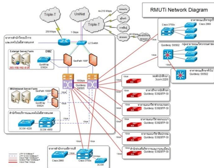
ภาพที่ 2 - 2 แสดงผังการเชื่อมต่อระหว่างอาคารหลักภายในศูนย์กลางมหาวิทยาลัย
